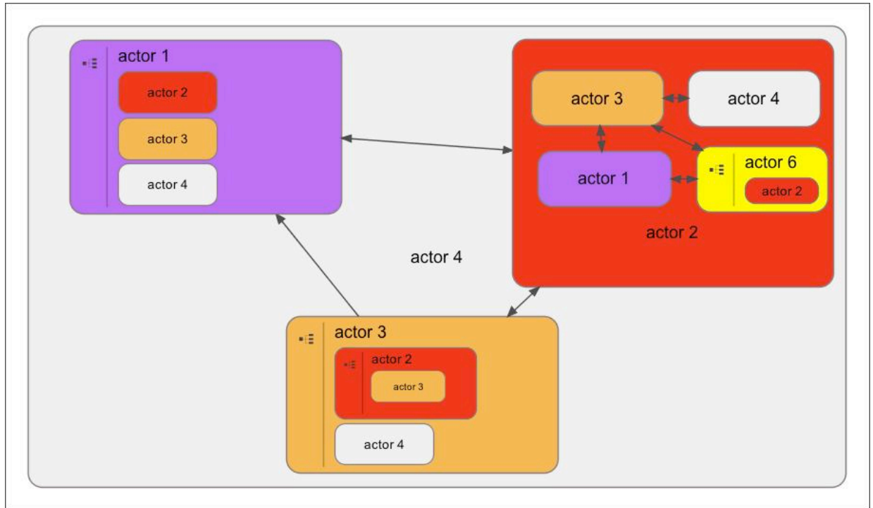
Afbeelding 1: Actor-netwerk
